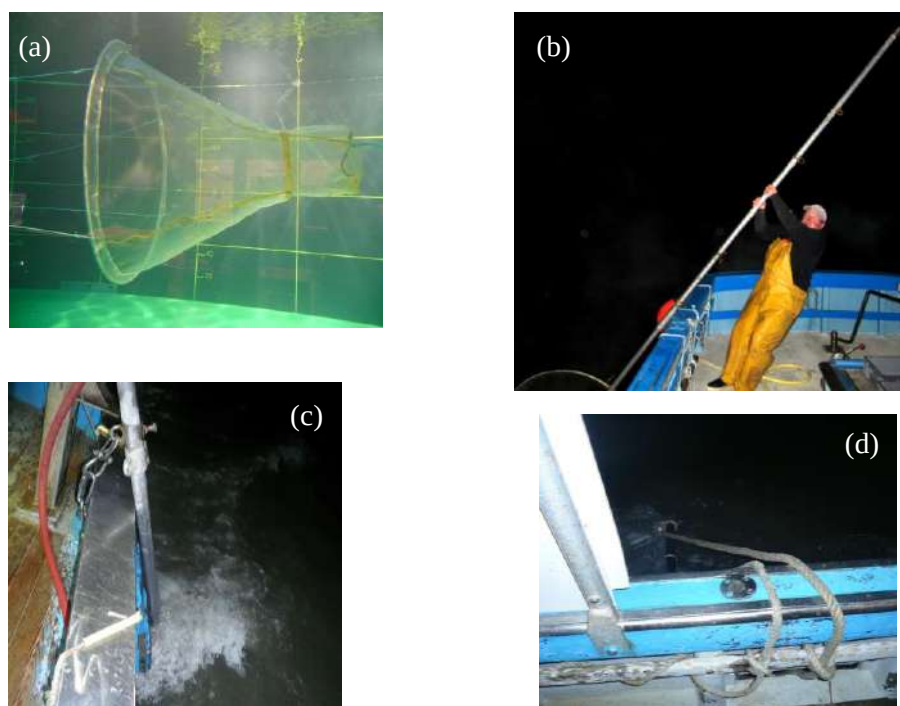
Figure 8 : Tamis et des systèmes de relèvement utilisés en Loire et en baie de Bourgneuf : (a) tamis de Loire immergé au bassin Ifremer de Boulogne s/ mer, (b) relèvement d'un tamis en Loire, (c) système d'accroche du tamis en Loire et (d) système d'accroche du tamis en baie de Bourgneuf
